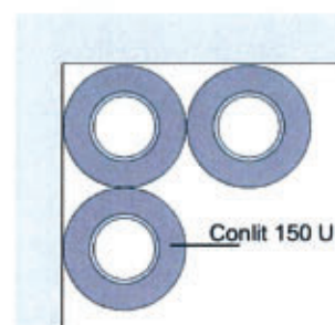
Prinzipskizze für Abstandsregelung bei Wand
